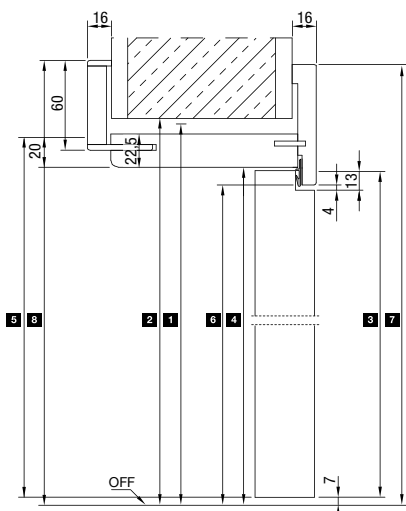
Вертикален разрез
