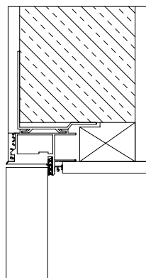
Хоризонтален разрез с врата без фалц
