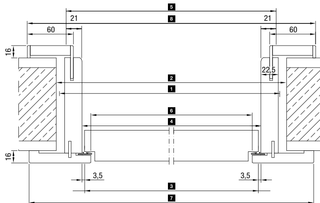
Хоризонтални разрези
